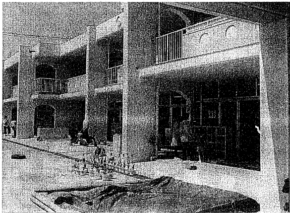
平成11年度から実施。外装改修や玄関、トイレのバリアフリー化の整備など大規模改修を行った八幡第四幼稚園園舎
