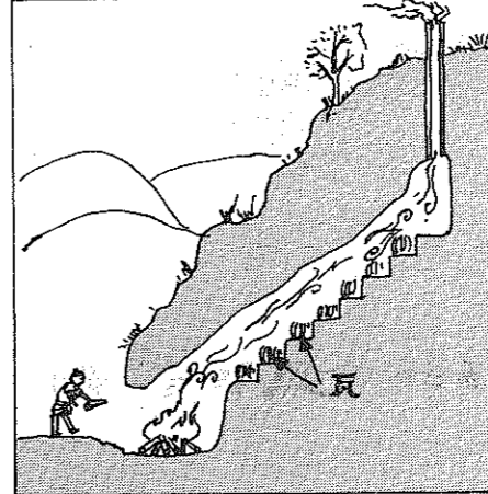
登り窯の模式図
