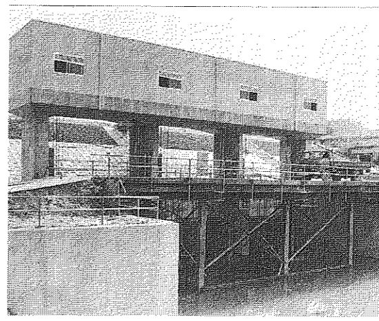
完成した樋門。ゲートを開けば一挙に内水を排除できる
