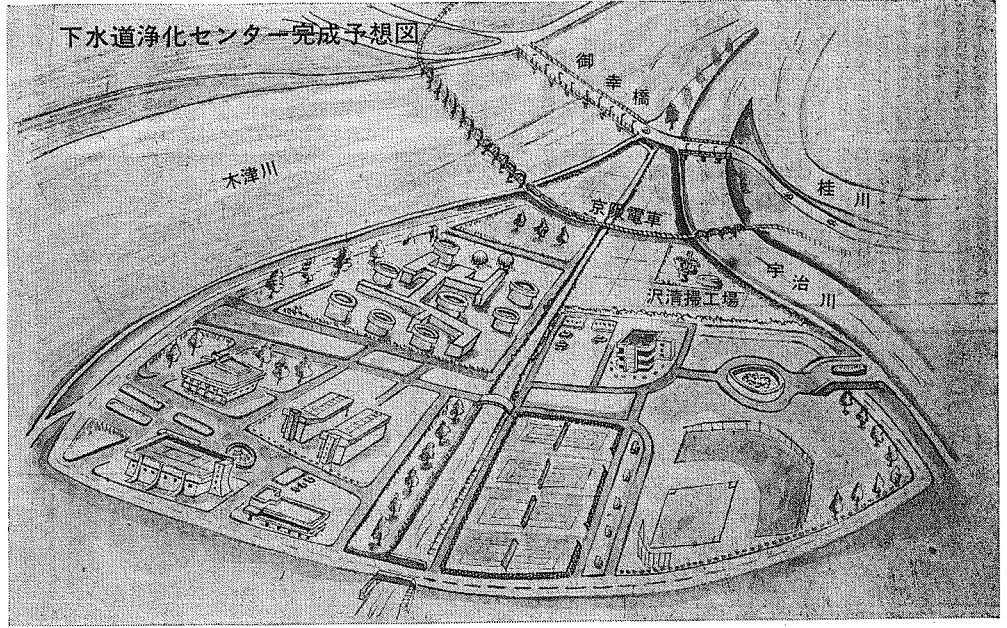
下水道浄化センター完成予想図
