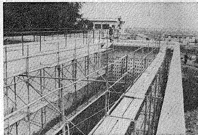
上水道の安定供給をめぐり着々と進められている第五期拡張工事（写真は取水井築造工事）
